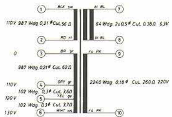
Netztrafo TK 14 BV 9005-531
