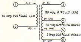
Oszillatorspule TK/TS 23 BV 9281-097
